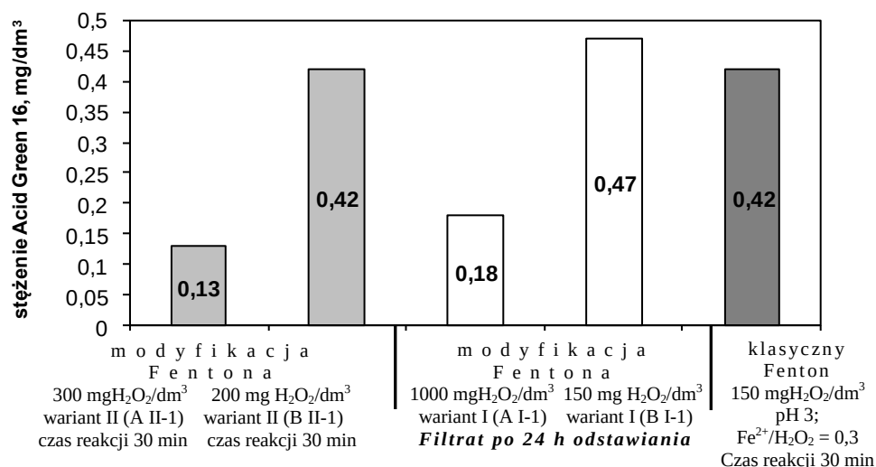
Rys. 4. Efekty odbarwiania przy zastosowaniu zmodyfikowanego oraz klasycznego odczynnika Fentona dla najkorzystniejszych dawek \text{H}_2\text{O}_2 (alkalizacja ścieków po procesie Fentona do pH 9)
