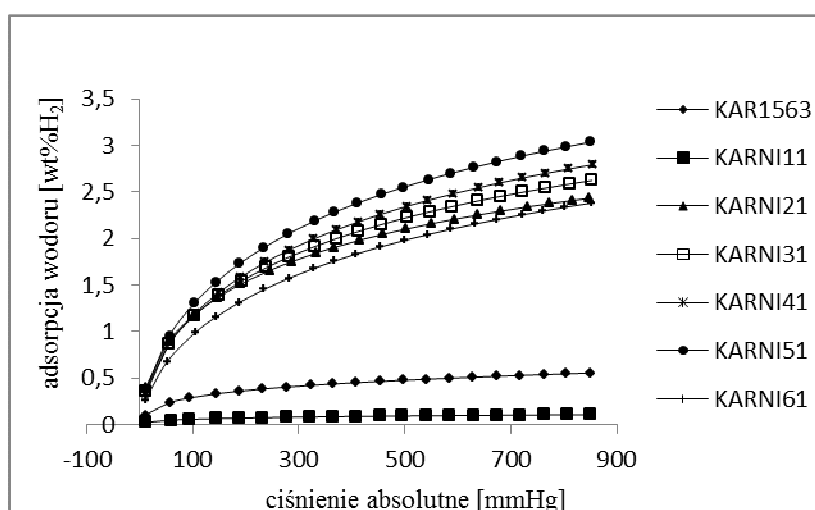
Rys. 7. Izotermy adsorpcji wodoru w temperaturze 77 K dla węgli KARNI11, KARNI21, KARNI31, KARNI41, KARNI51, KARNI61
