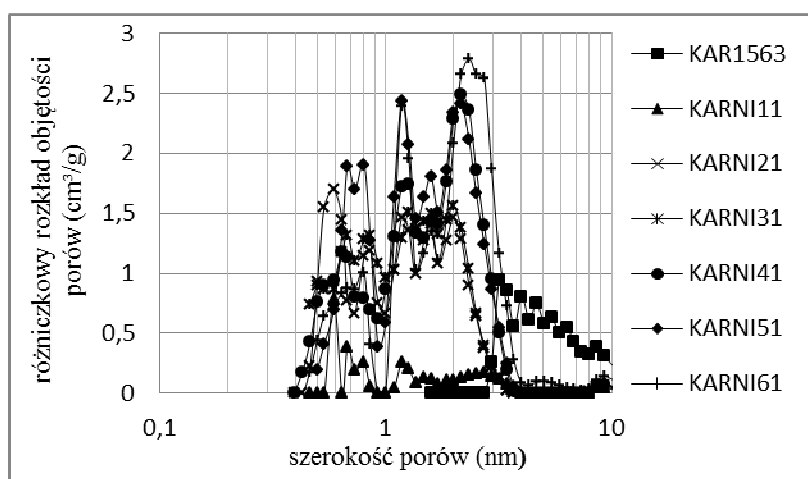
Rys. 6. Wykres zależności różniczkowego rozkładu objętości porów w funkcji szerokości porów dla karbonizatu KAR1563 oraz serii węgli KARNI11 - KARNI61
