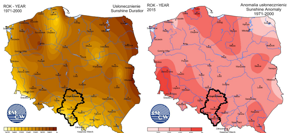
Rys. 8. Mapy klimatu Polski (z wyróżnionym obszarem województwa śląskiego): usłonecznienie z wielolecia 1971-2000 i anomalia usłonecznienia w 2015 r., na podstawie [10]
