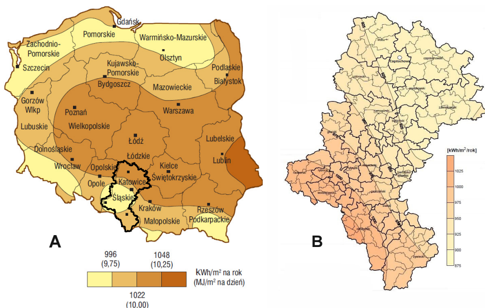
Rys. 2. Potencjał energii promieniowania słonecznego w województwie śląskim: A [5], B [6]
